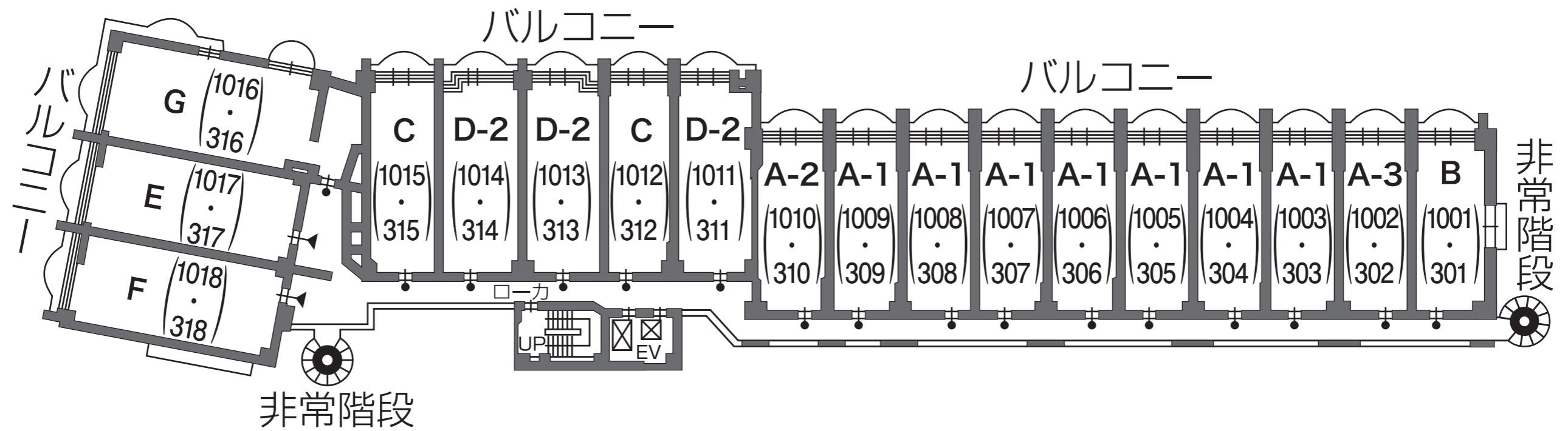
3~10階平面図
