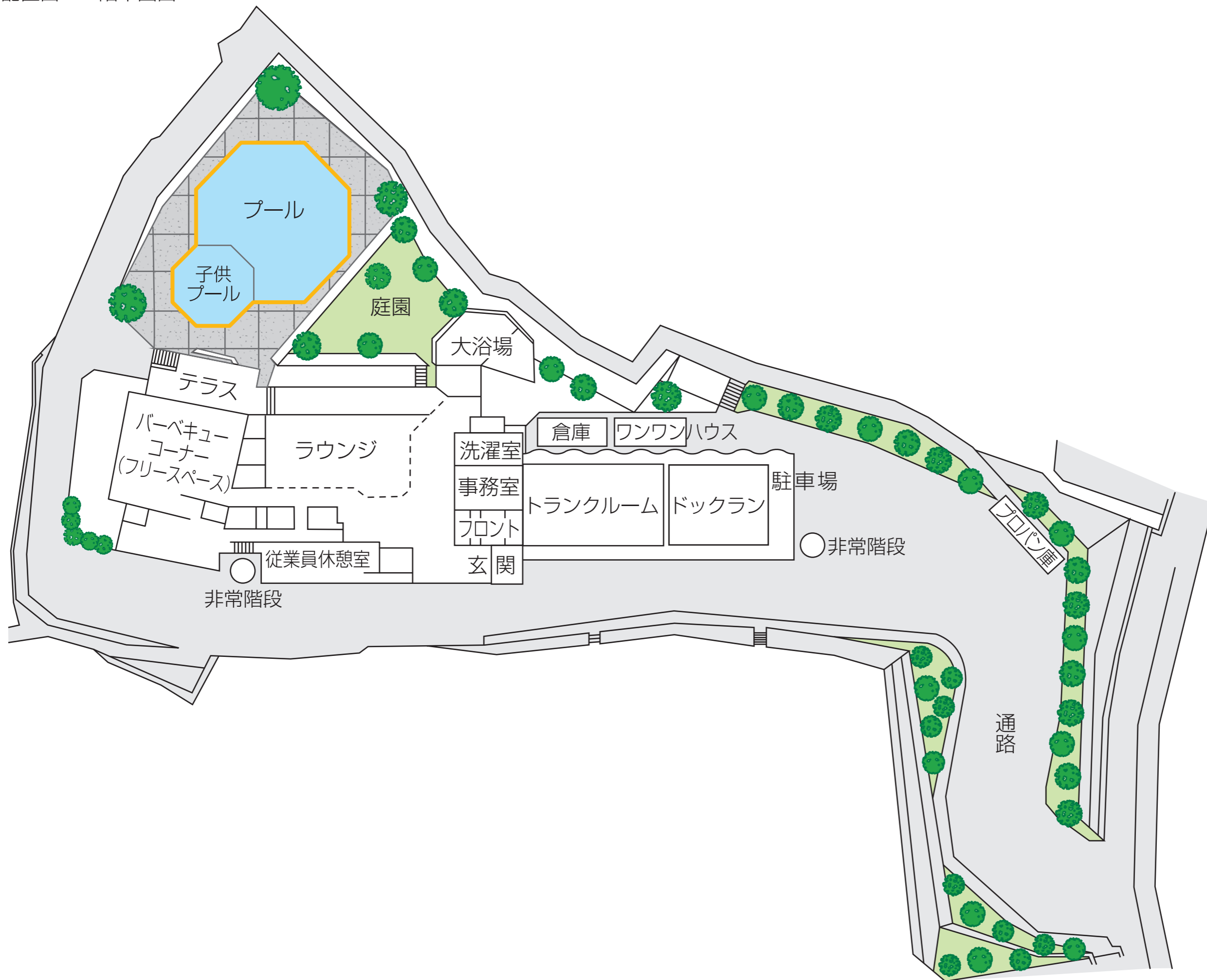
敷地配置図・1階平面図
